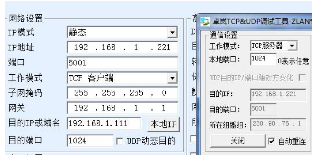
图 20 串口服务器作为客户端
