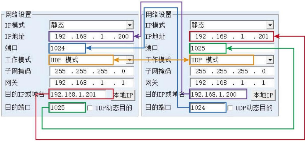
图 28 UDP 设备对联参数配置
