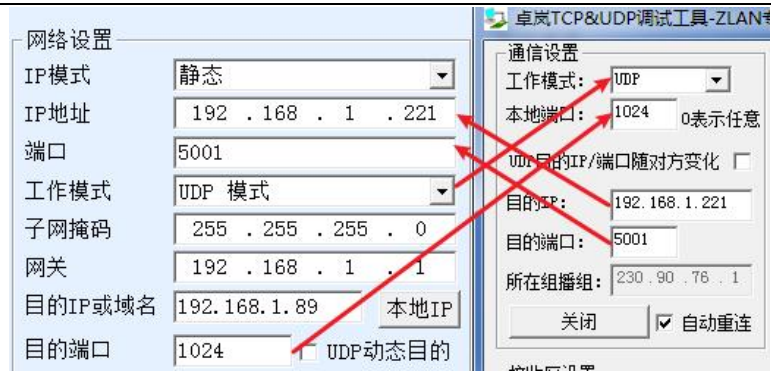
图 25 UDP 模式参数配置
