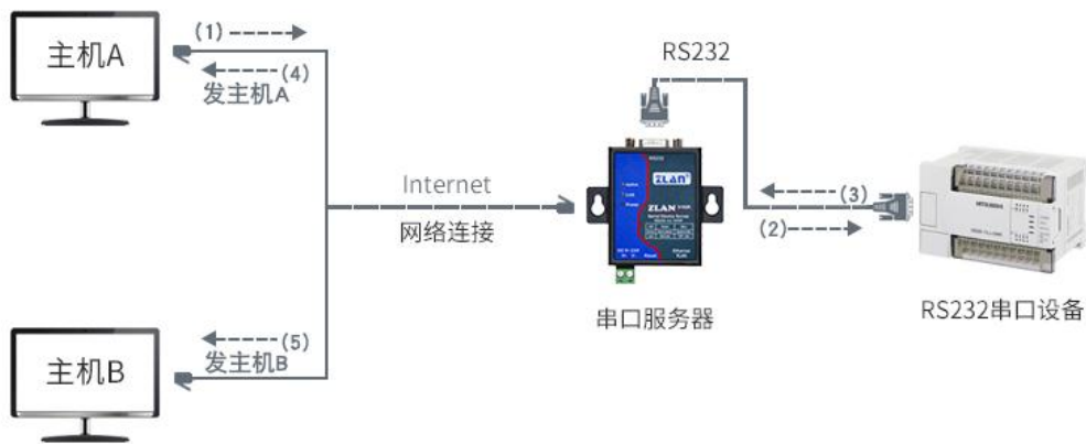
图 36 多主机功能演示
