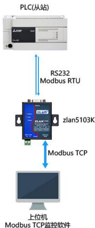
图 34 存储型 Modbus 网关工作方式
